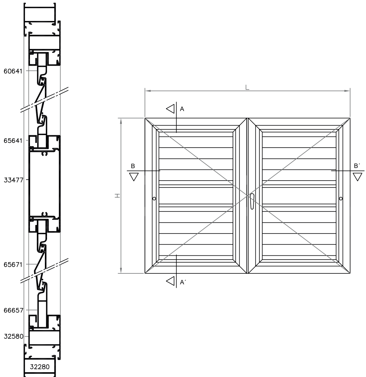
SECCIÓN A-A'
