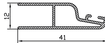
LAMA COMPENSADORA 41 66641
