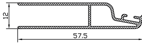
LAMA COMPENSADORA 57.5 66657
