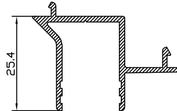
PERFIL COMPENSADOR 65640
