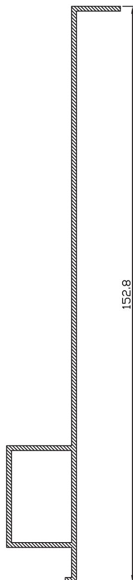
PREMARCO OBRA 152.8 52501
