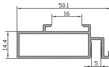
PREMARCO 50 ALUPLAVER 52538
