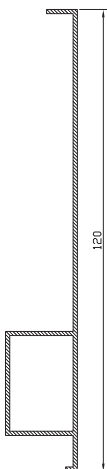
PREM. OBRA 120 52505
