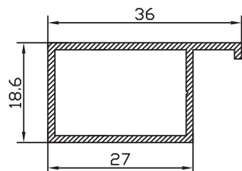
PREMARCO OBRA 36 52506
