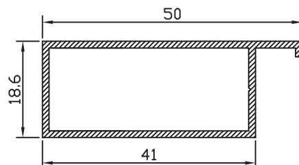
PREMARCO OBRA 50 52507
