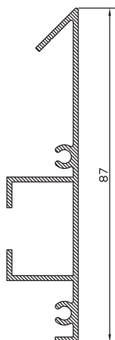
PREM. OBRA 87 52544
