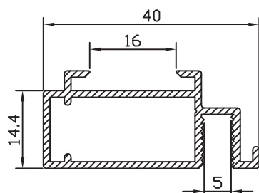
PREMARCO 40 ALUPLAVER 52542
