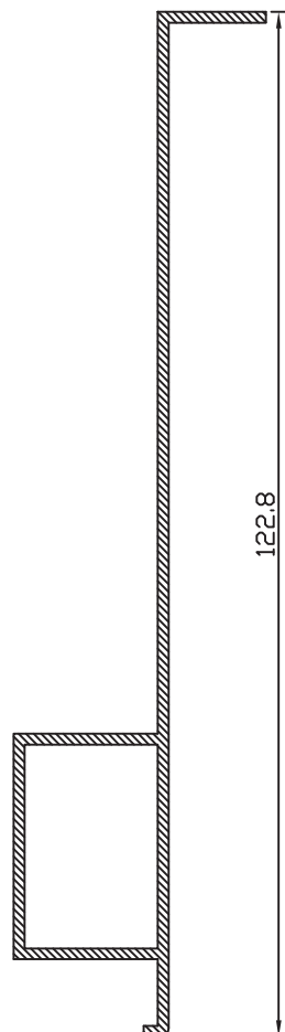
PREM. OBRA 122.8 52502
