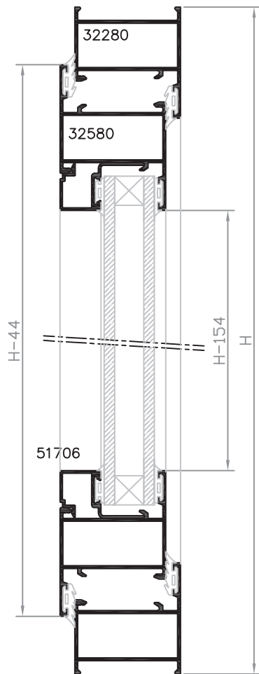
SECCIÓN A-A'
