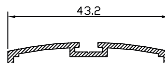
DOBLE EFECTO 39099
