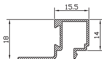
JUNQUILLO CAMARA 21.2 51706
