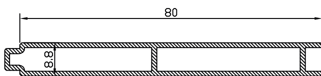
LAMA MACHIHEMB.80 60676
