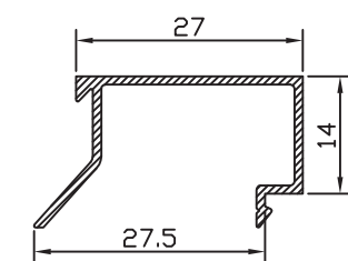
JUNQUILLO CAMARA 9.7 51702
