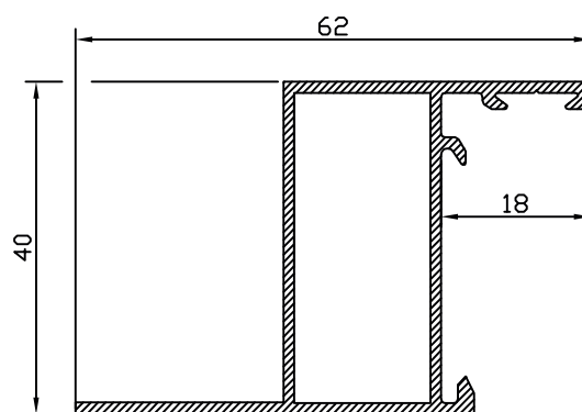
MARCO CON PREMARCO 32283
