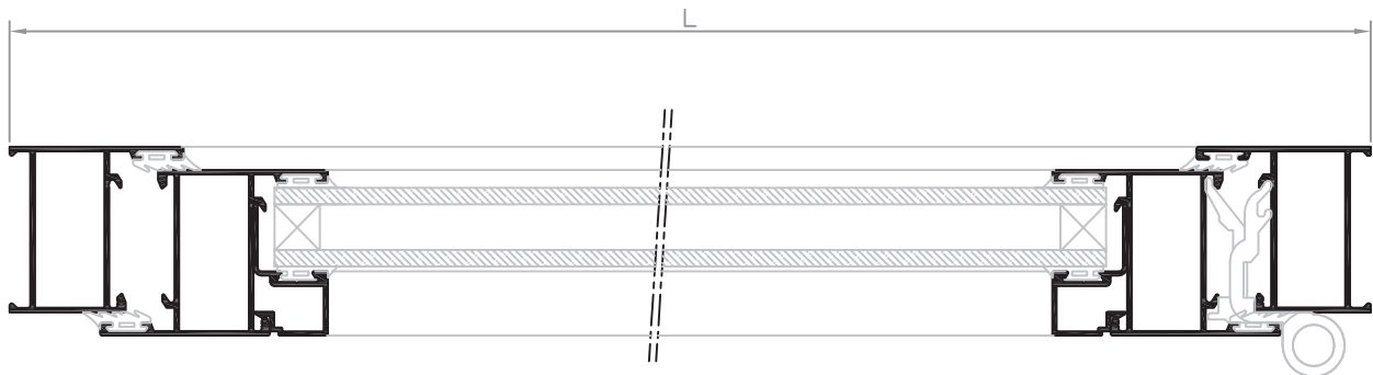
SECCIÓN B-B'
