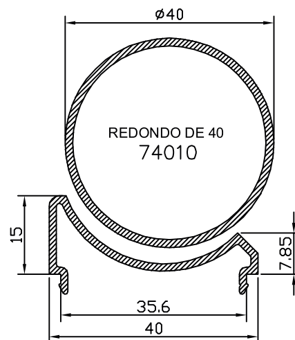
REDONDO DE 40 74010
