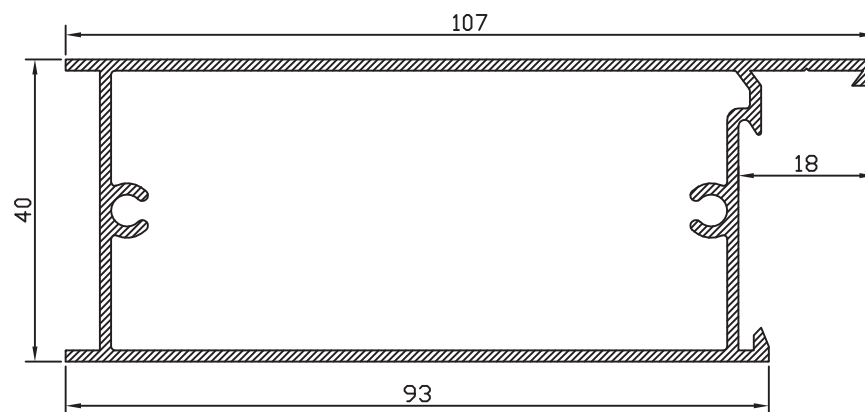
ZÓCALO MARCO 33476
