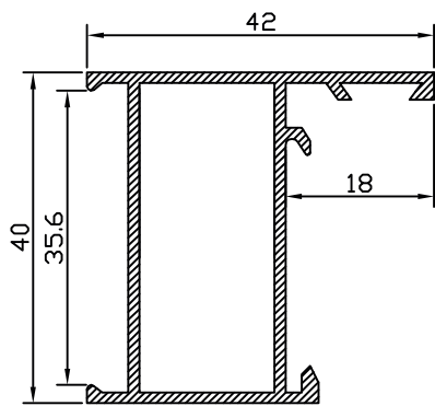
MARCO 32280
