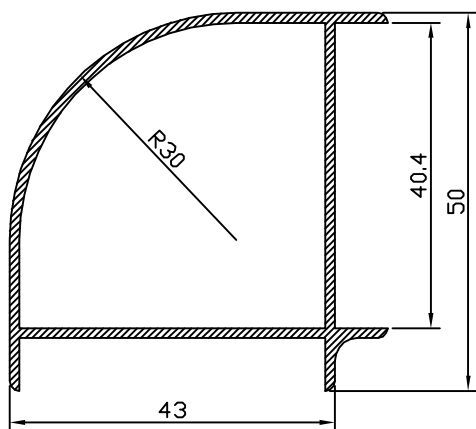
ESQUINERO 90° 33092
