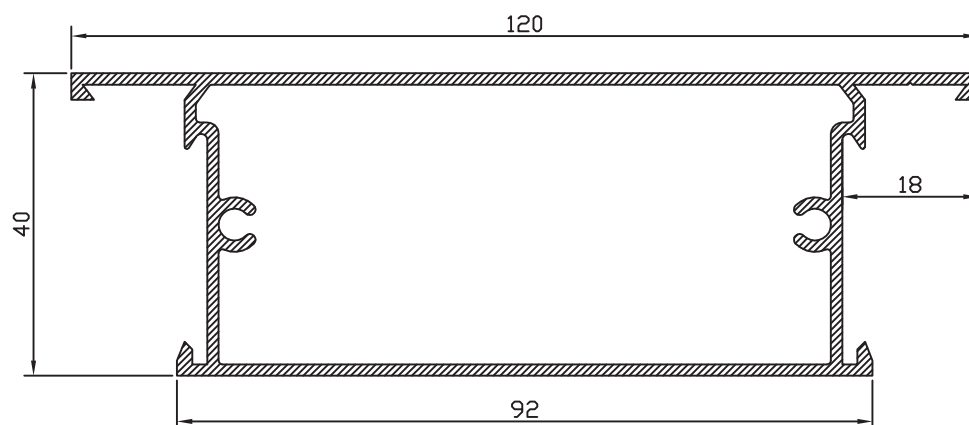
ZÓCALO INTERMEDIO 33477
