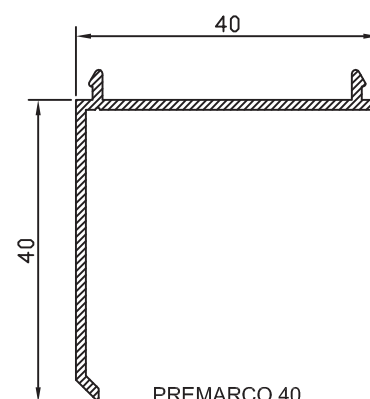
PREMARCO 40 28101
