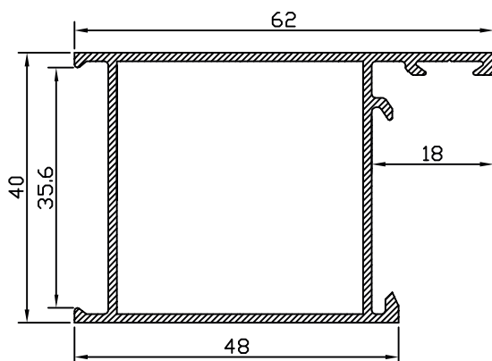
MARCO PUERTA 33280
