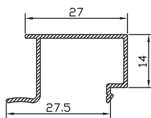
JUNQUILLO CAMARA 9.7 51720
