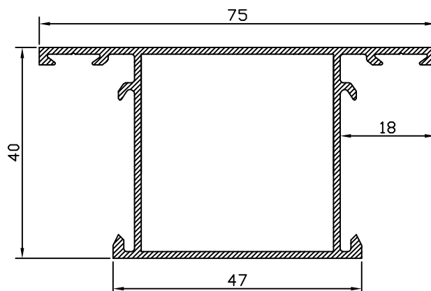
PILASTRA 75 33580
