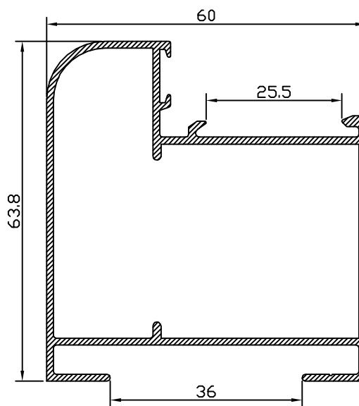
MARCO ESCAPARATE 33282
