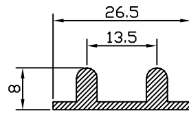
MARCO INFERIOR VITRINA 82303
