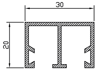
MARCO SUPERIOR VITRINA 82302
