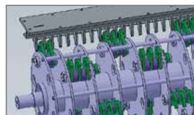
Sistema di taglio con incrocio coltello e controcoltello Cutting blade runs into the counter-blade Schnittsystem Messer-Gegenmesser Sistema de corte con cruce de cuchilla y contra cuchilla Système de coupe avec croisement couteau et contre couteau
