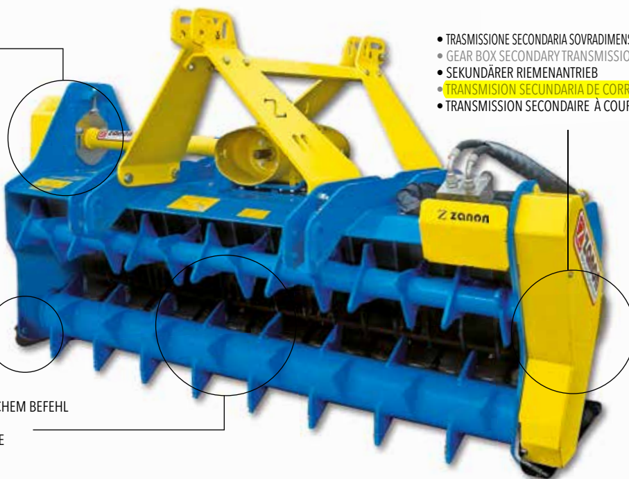
Sistema di taglio con incrocio coltello e controcoltello Cutting blade runs into the counter-blade Schnittsystem Messer-Gegenmesser Sistema de corte con cruce de cuchilla y contra cuchilla Système de coupe avec croisement couteau et contre couteau
