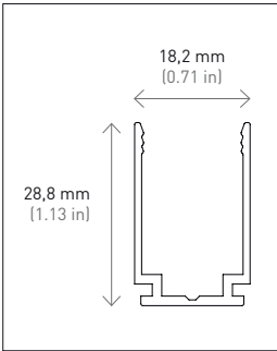
Aluminium guide profile. Perfil guía aluminio.
