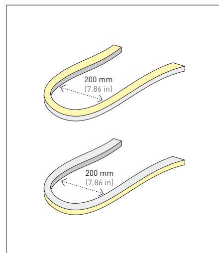
Bending diameter 200 mm. Diámetro de curvatura 200 mm.
