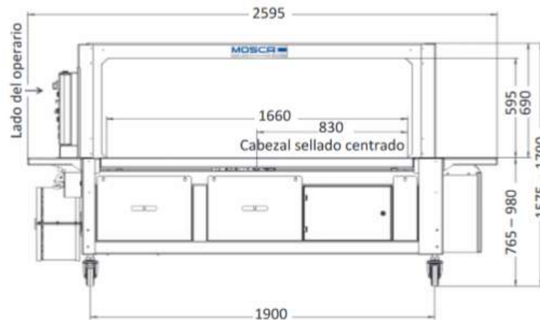
Esquema RO-MC-6 / 1650 x 600 mm
