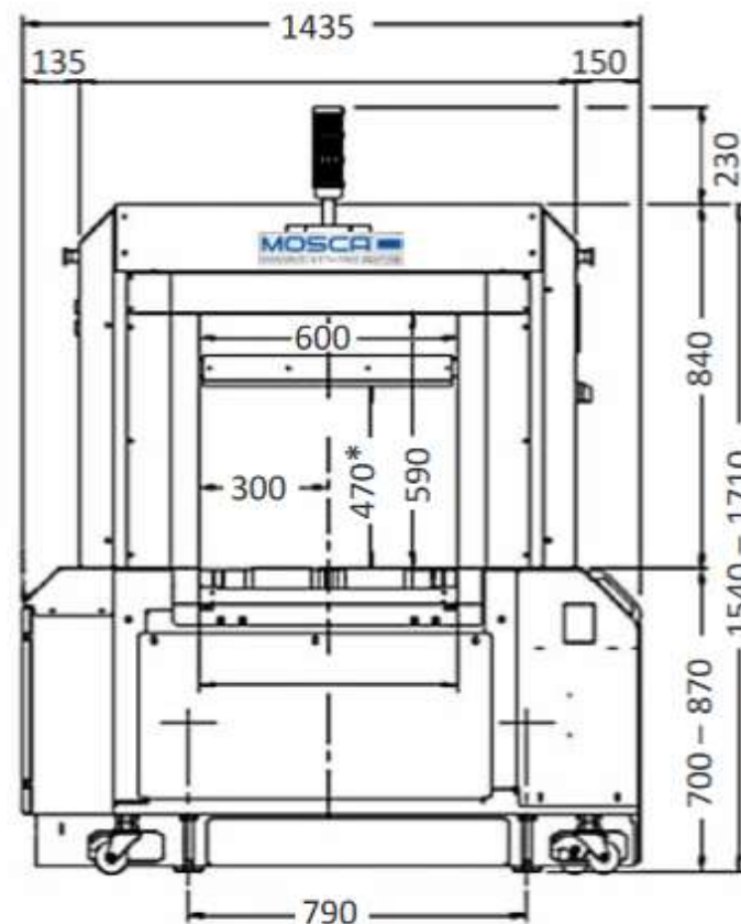
*400 mm del pisón neumático
