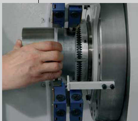
Particolare regolazione camme Cams setting detail
