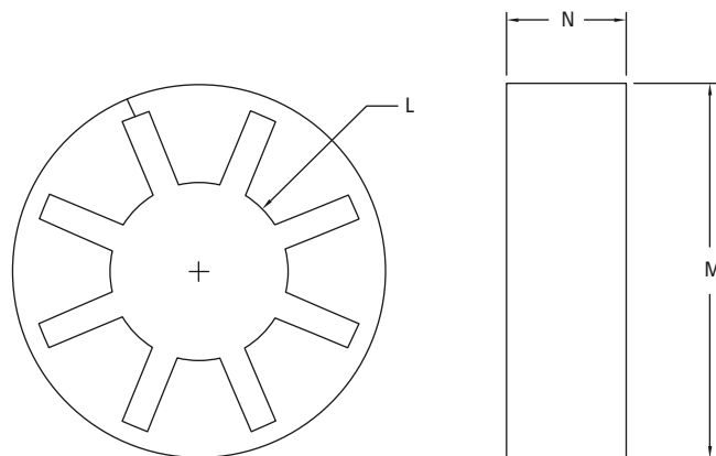
Fig. 16. Quick-Flex insert.
