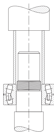
Fig. 11. Arbor press method.
