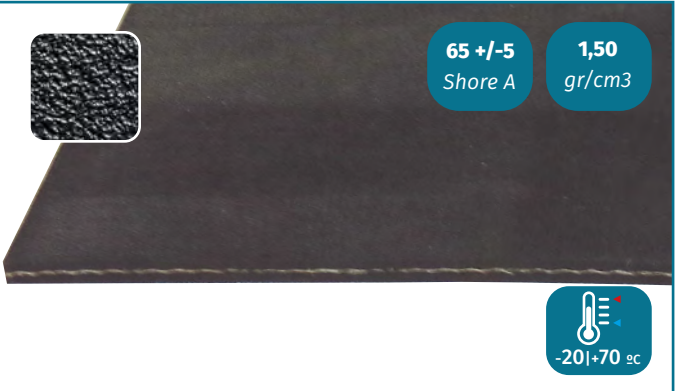
NR-SBR Goma Común Rugosa con 1 Inserción Textil SBR rough rubber with 1 textile insertion
