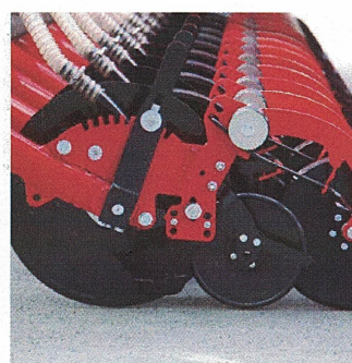
Rueda de presión en la ranura de siembra
