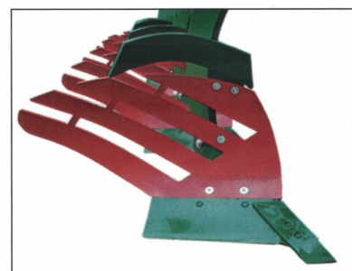
Detalle teja de láminas "TL"
