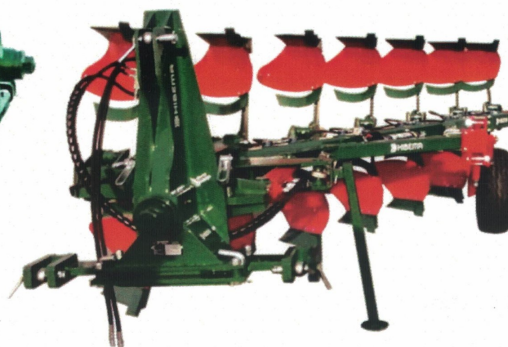
Kit cierre del arado a partir de 6 cuerpos
