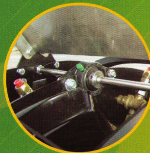
Sistema oscilante del efecto tornado Oscillating system of the returned effect Système oscillant de l'effet tornade
