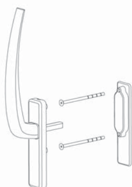
4 Manilla interior con uñero exterior
