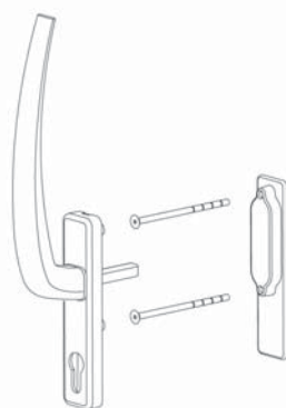
/a Manilla interior con entrada para cilindro
