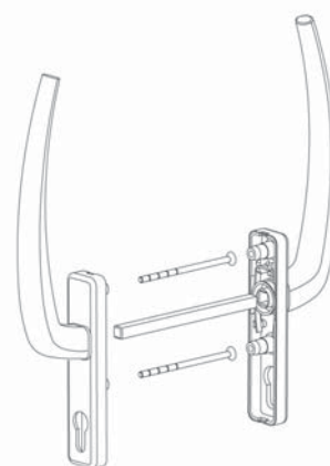
/b Manilla doble con entrada para cilindro
