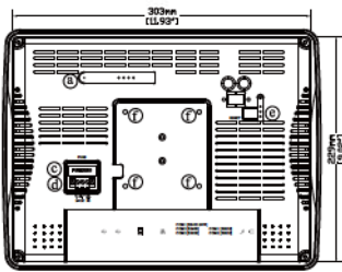
Vista Posterior
