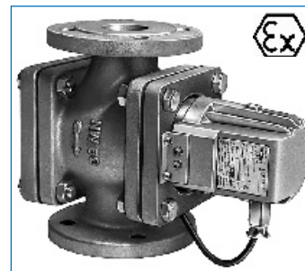
Mirillas para conducciones con o sin iluminación
