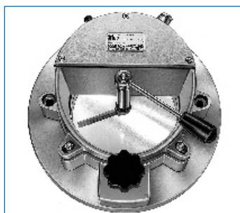
Mirillas practicables de apertura roscada tipo KSG(B) con o sin proyector incorporado
