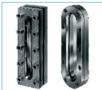
Mirillas (niveles) con extremos rectangulares RSG (R, RR) y redondeados LSG (R, RR)
