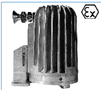
Proyectores CHEMLUX serie 20/45/100 en ejecución Ex y no Ex hasta 100 W, T4
