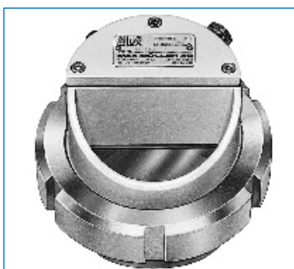
Proyectores tipo HLM(R) para mirillas roscadas similares a DIN 11851
