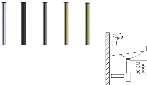
Alargadera para sifón. Bottle trap extension.
