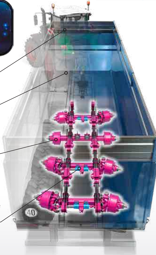
Cilindro dualfunction, per ogni tipo di sterzante Dual Function cylinder, for each steering axles Dual-Funktionszylinder für jede Lenkachse
