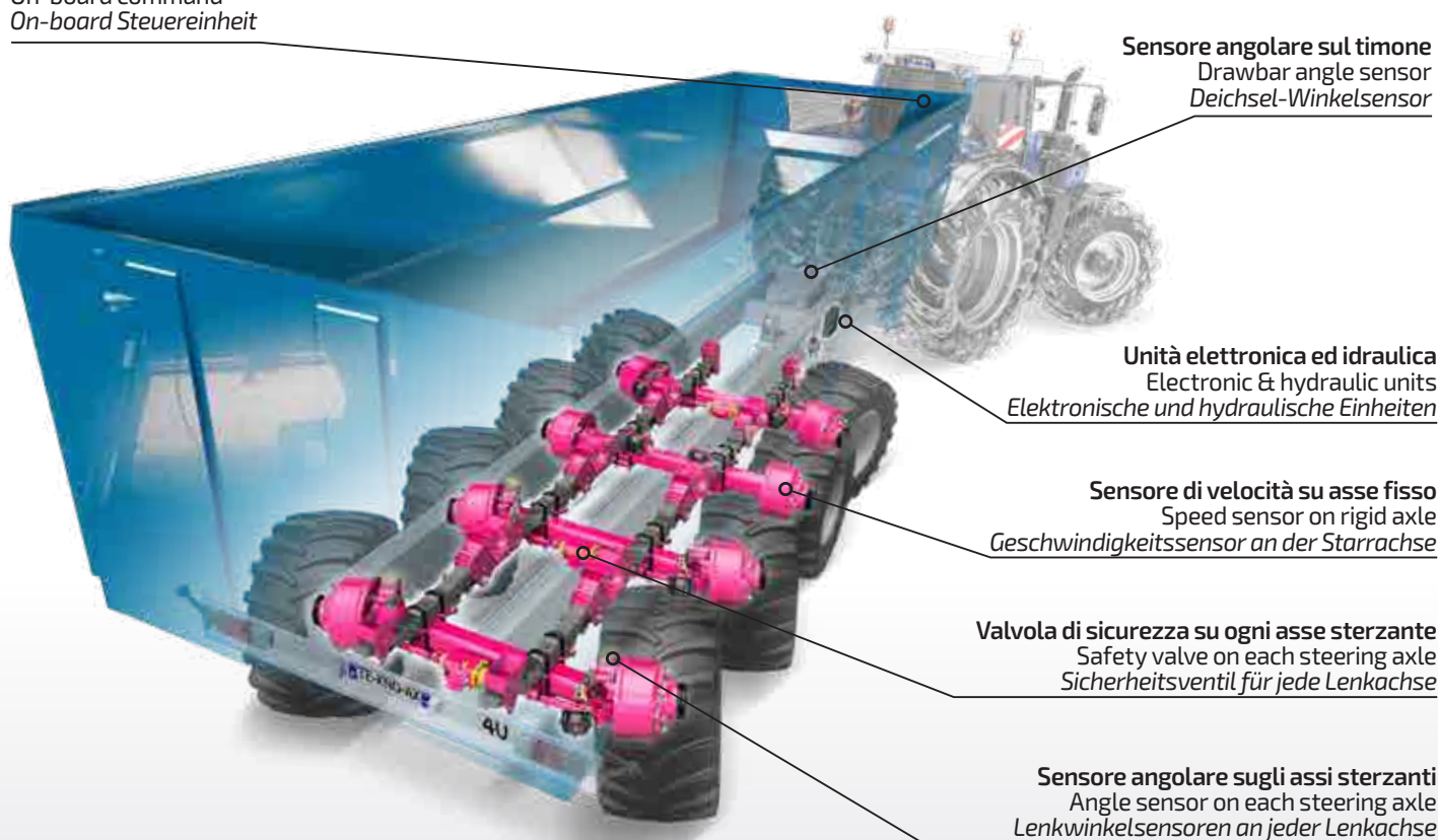
Pannello di controllo On-board command On-board Steuereinheit
