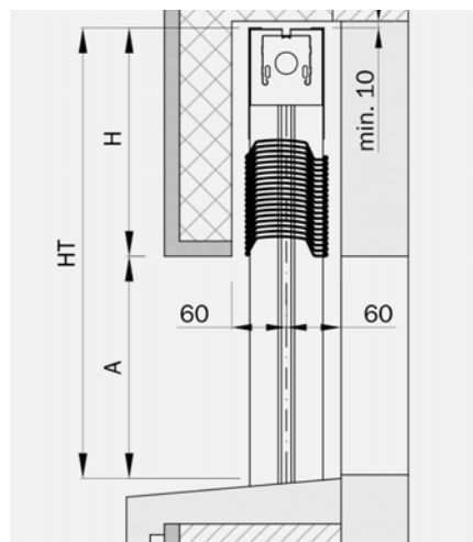
Sección vertical.
