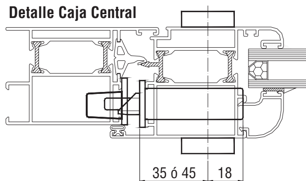
Motor eléctrico (Fresado en hoja; 310x16x60) Ref. K-18153-01-0-0
