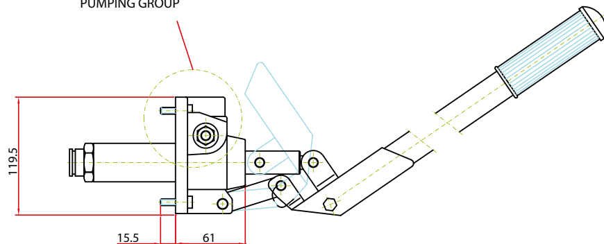
GRUPO DE BOMBEO PUMPING GROUP
