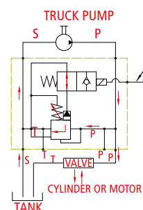
Con limitadora With Relief Valve
