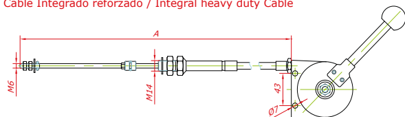
Cable Integrado reforzado / Integral heavy duty Cable
