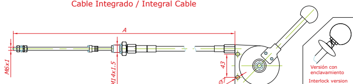
Cable Integrado / Integral Cable
