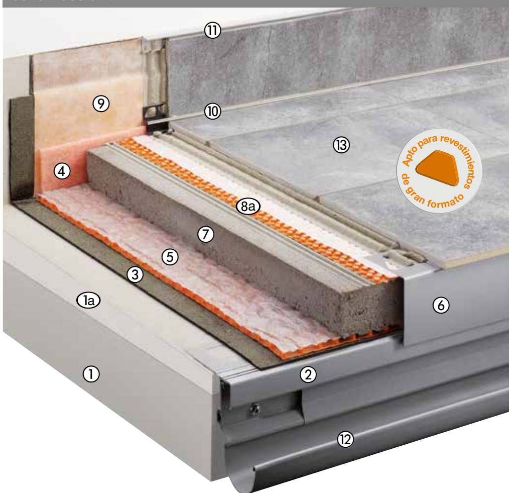
CONSTRUCCIÓN 5A
