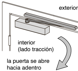
MONTAJE EN PUERTA, LADO TRACCIÓN
