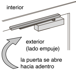
MONTAJE EN PUERTA, LADO EMPUJE
