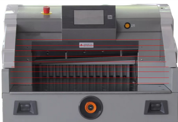
Barreras inmateriales de seguridad
