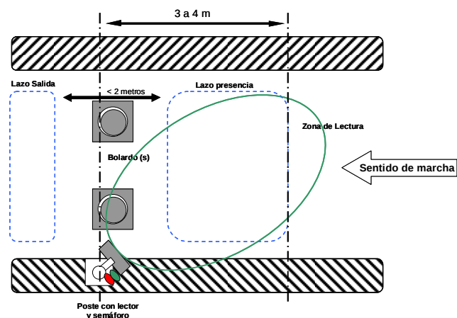
Vía con bolardos y Teletag
