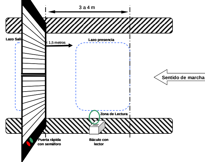
Vía con puerta rápida y lector de proximidad
