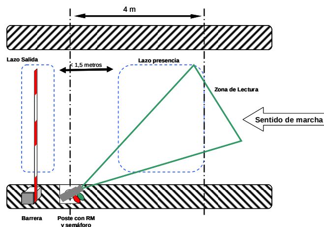
Vía con barrera y reconocimiento de matrículas
