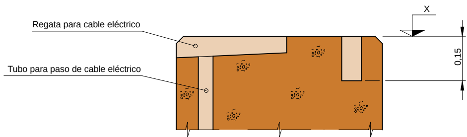
SECCION "A-A"
