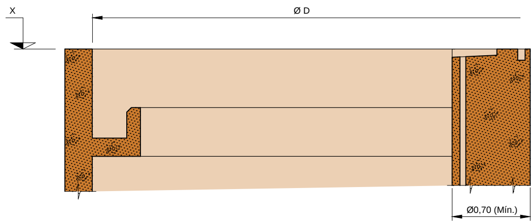
SECCION "A-A"
