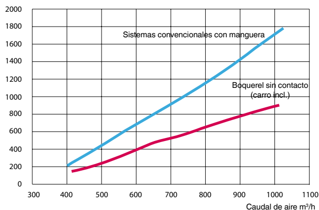
Caída de presión Pa
