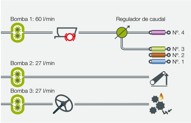
Circuito hidráulico de 3 bombas con un rendimiento hidráulico total de 114 l/min: 87 l/min para los distribuidores hidráulicos y el elevador trasero y 27 l/min para la dirección y los engranajes.
