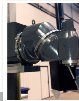
REPARACIÓN DE CABEZALES AUTOMÁTICOS Y MANUALES
